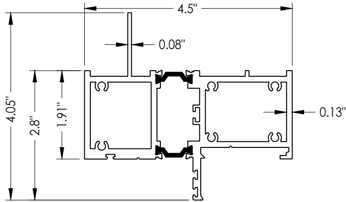
10 FRAME (FIN)
